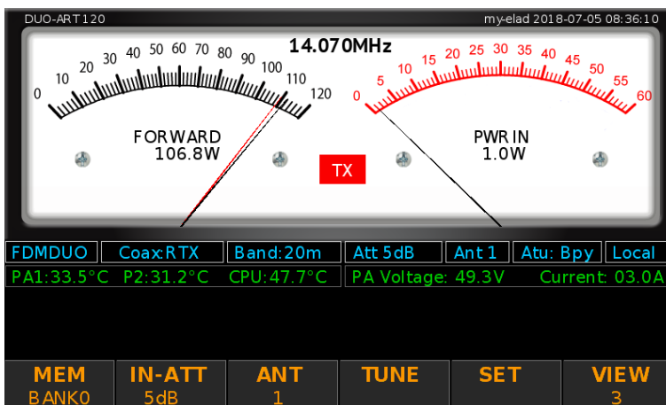
VIEW 3 : potenza diretta e potenza in ingresso.
