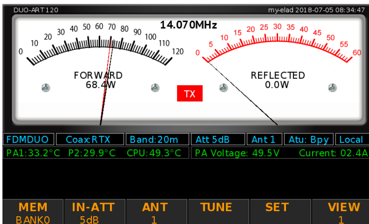
VIEW 1 : potenza diretta e potenza riflessa.
