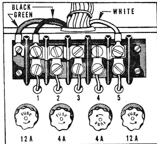
115 V.A.C.
