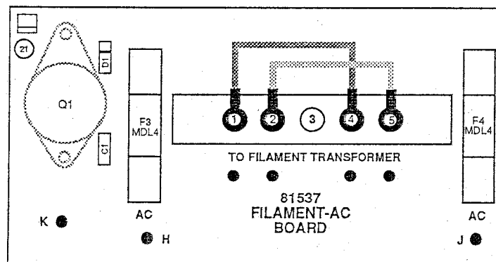
115 VAC WIRING
