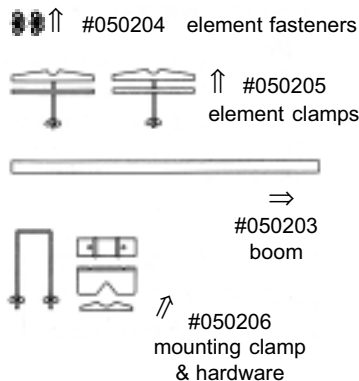
A502HB Parts List
