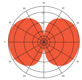
E-plane: 100 MHz
