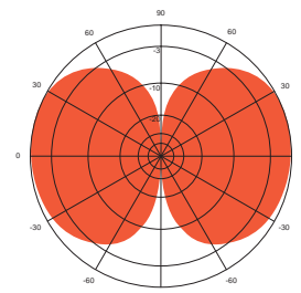
E-plane: 400 MHz
