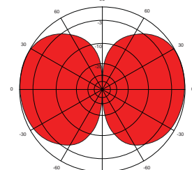
E-plane: 400 MHz
