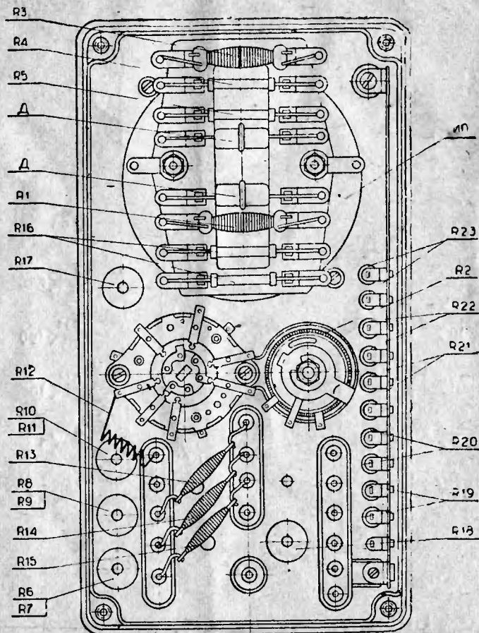
Д Расположение элементов схемы ампервольтметра типа Ц-20
