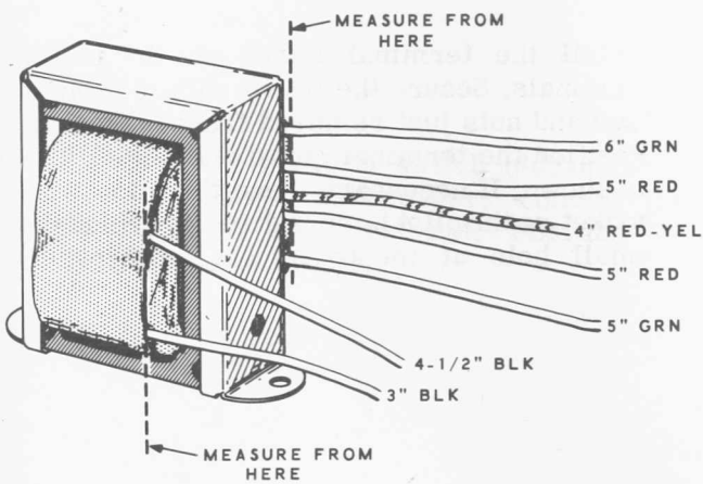
Detail 1E
