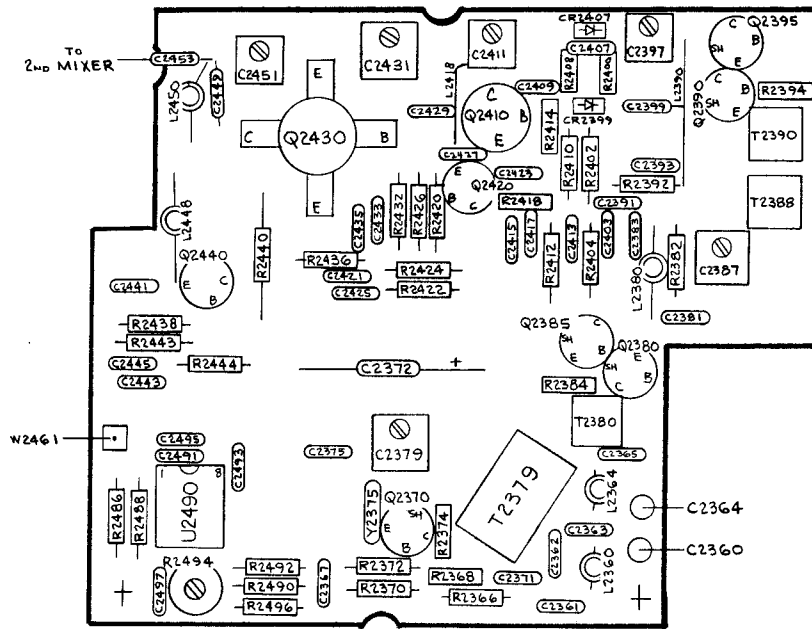
7L18 H-5033-02 A2360A1 500MHz LO
