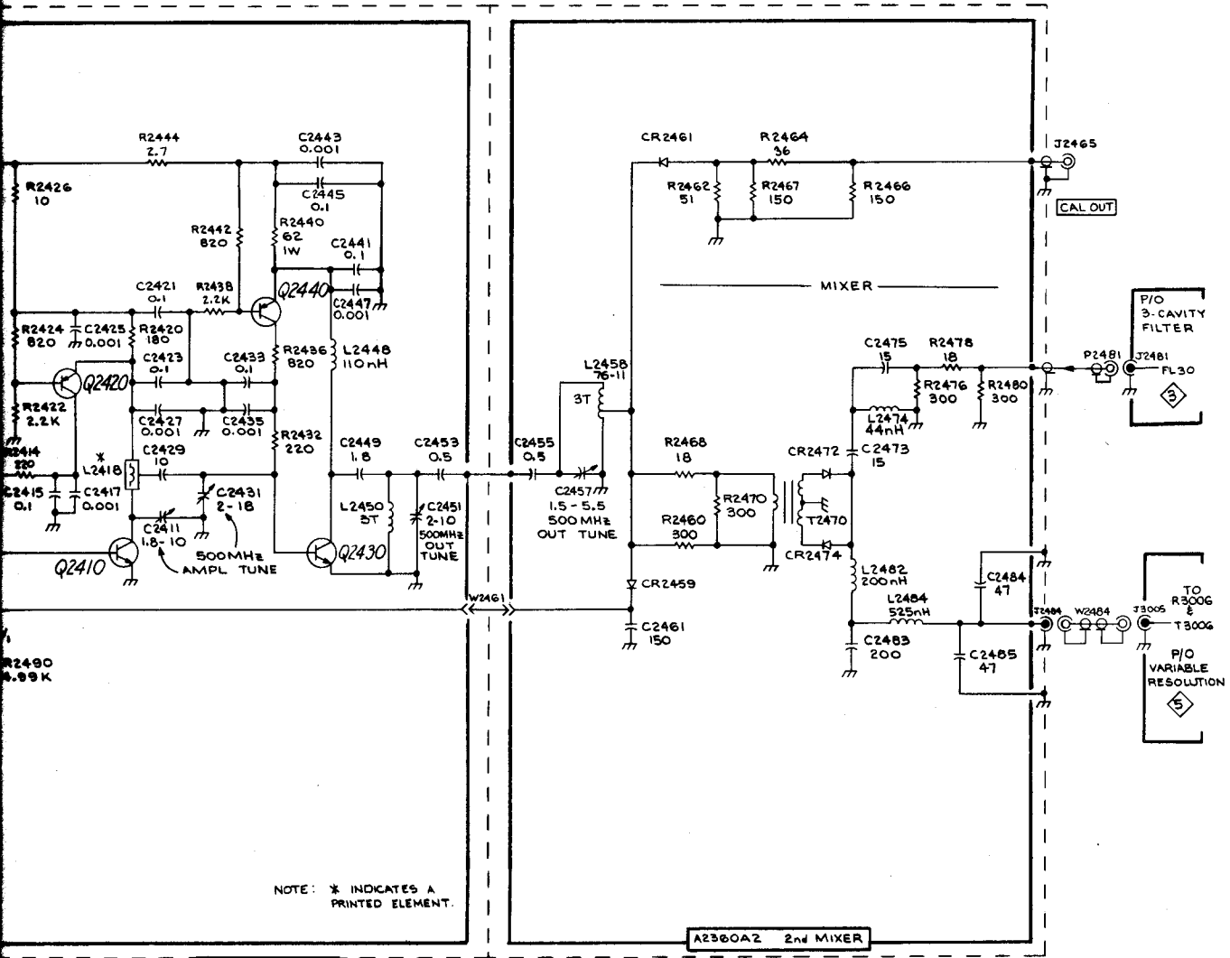
500MHz LO CHAIN & MIXER 4
