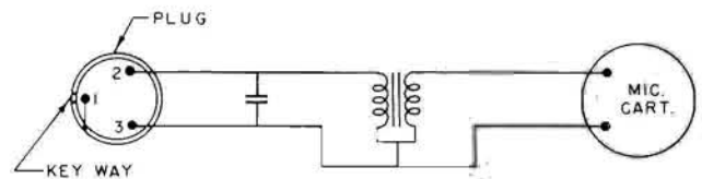
SCHEMATIC 10DA, 10DA-50, 10DA-500
