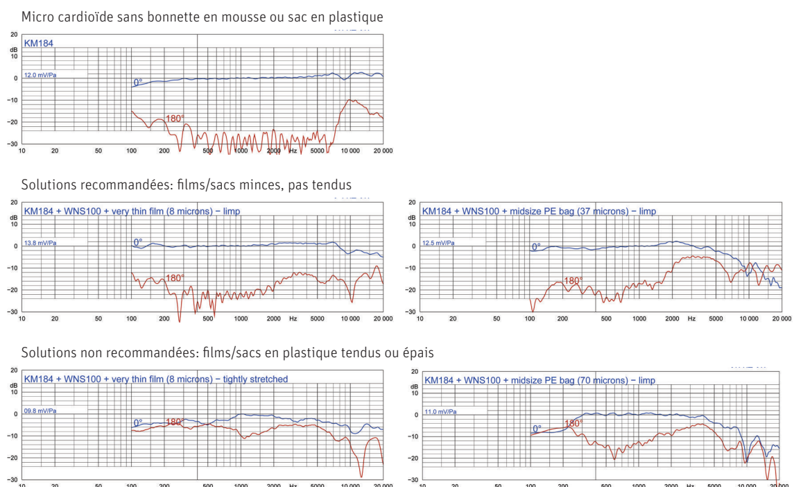
FIGURE 2: Exemples de mesures du KM 184 avec différentes configurations de sac en plastique et d'une bonnette WNS 100 (mesurées à 1 m)
