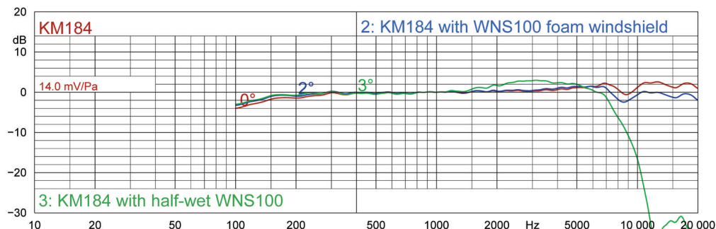
FIGURE 1: Réponse sur axe du KM 184, avec la bonnette WNS 100 (sec) et avec WNS 100 humide.
