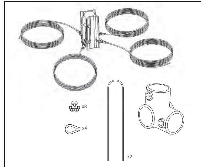
Fig. 3. Kit de torre de 27 pies (8,3 m)
