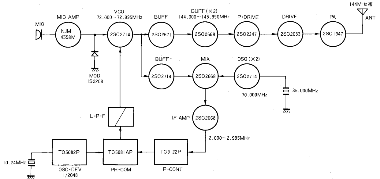
TH-21 送信機系統図
