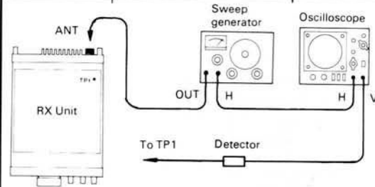
Fig. 20 RX 2. Helical
