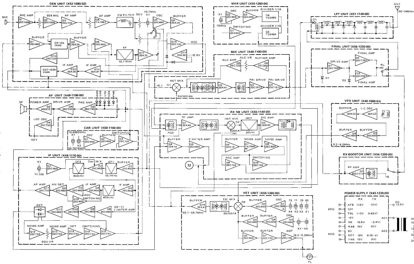
図11 TS-600ブロックダイアグラム
