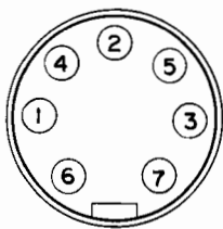
EXT CONT背面パネルから見た図
