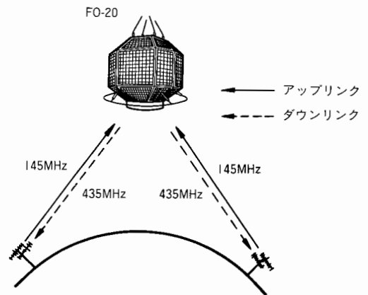
FO-20アナログ・モードの送受信周波数関係
