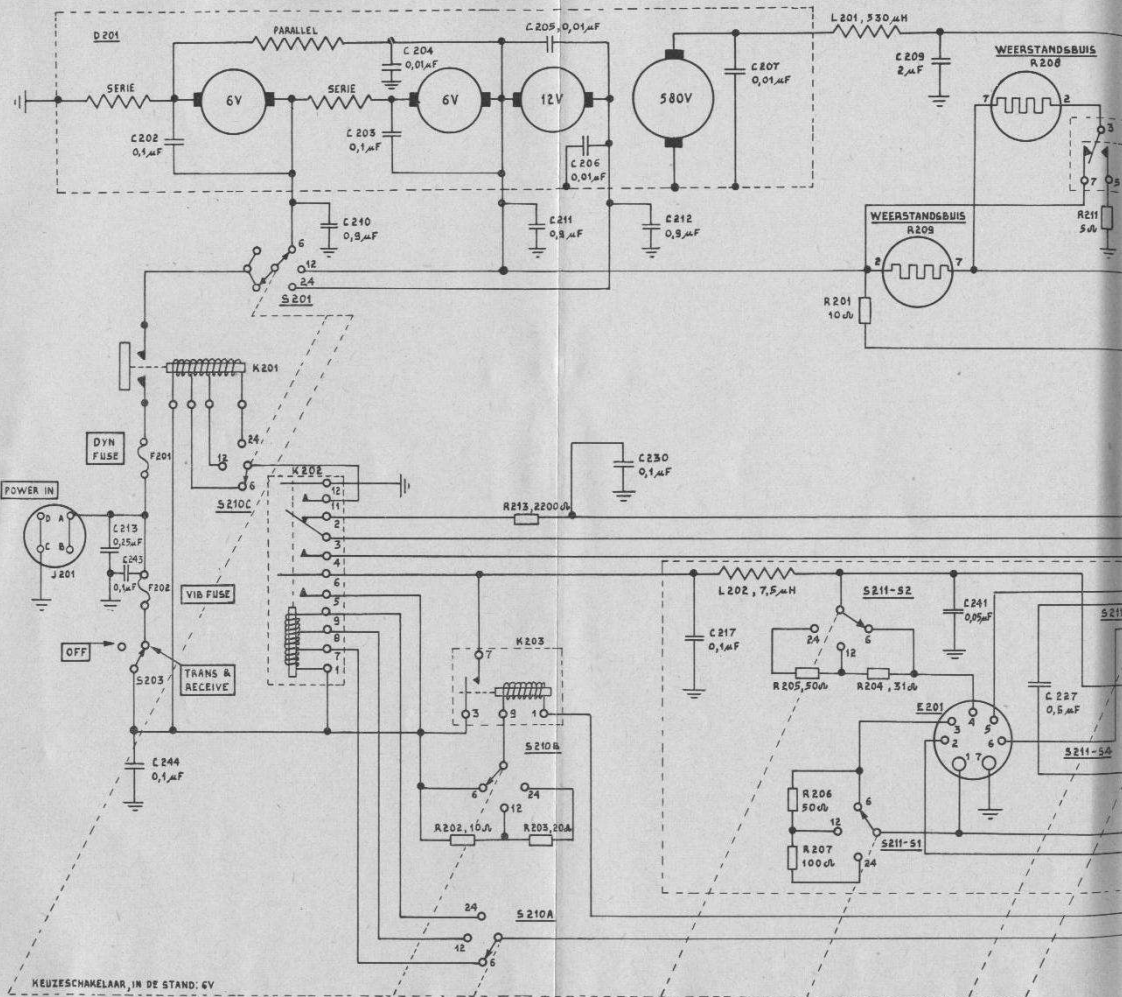
Fig. 77A. Voedingseenheid DY-88FR/GRC-9, prinsieschema
