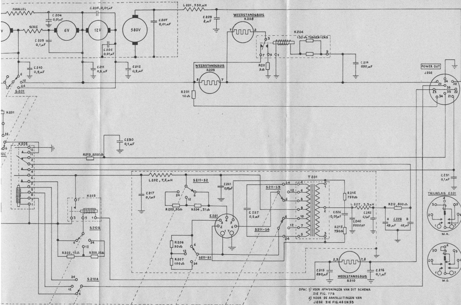
Fig. 77A. Voedingsenheid DY-88FR/GRC-9, prinseschema
