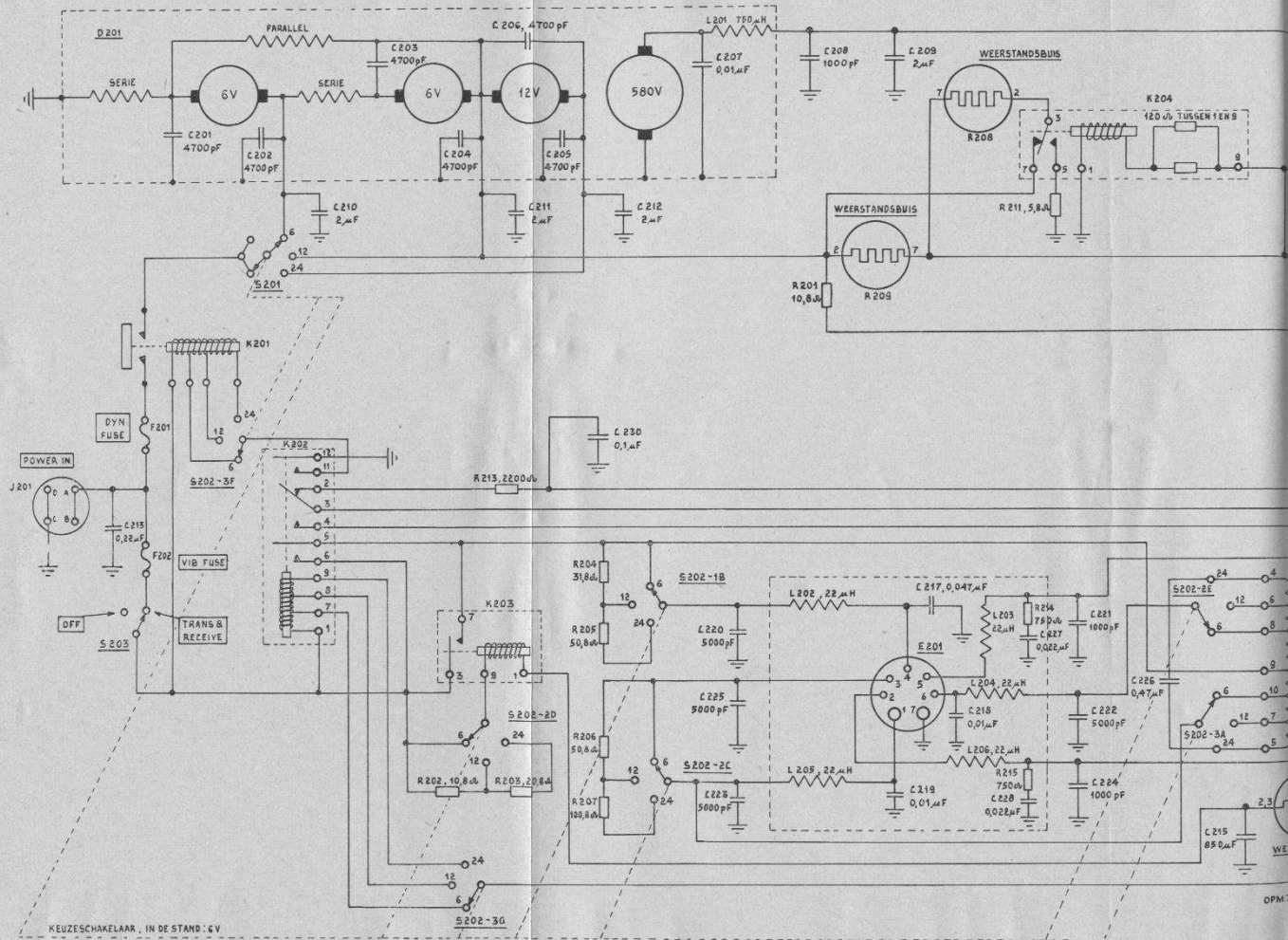
Fig. 77B. Voedingseenheid DY-88GY/GRC-9, prinsieschema
