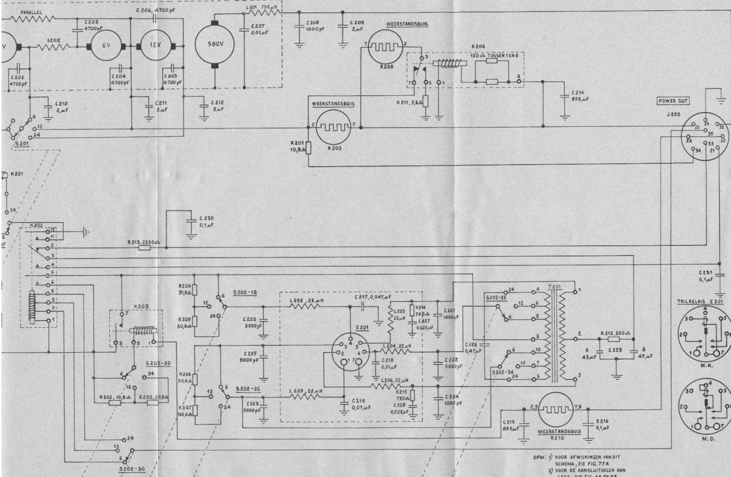
Fig. 77B: Voedingseenheid DY-88GY/GRC-9, prinsieschema
