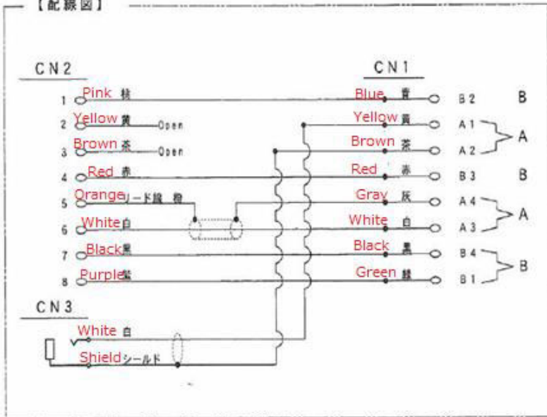
【配線図】
