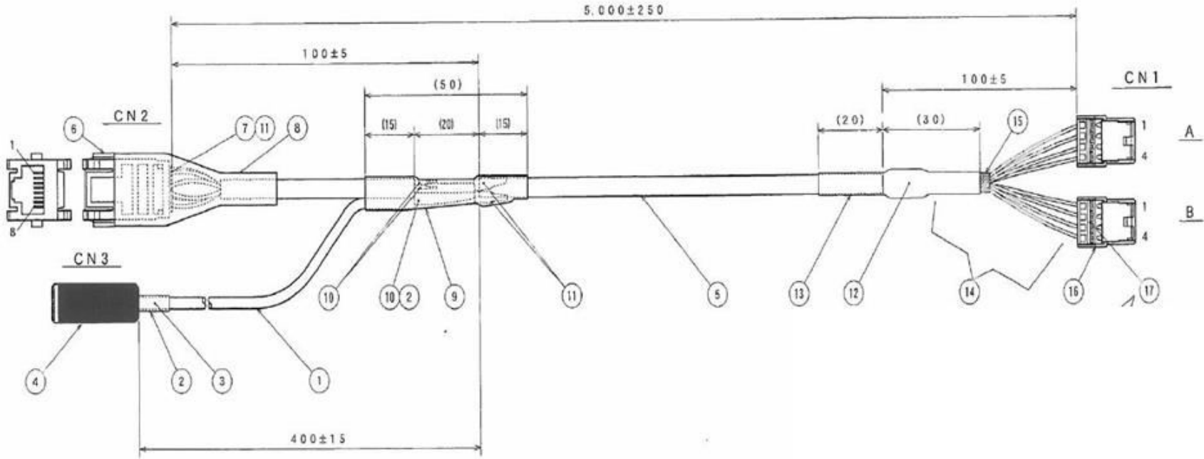
【配線図】
