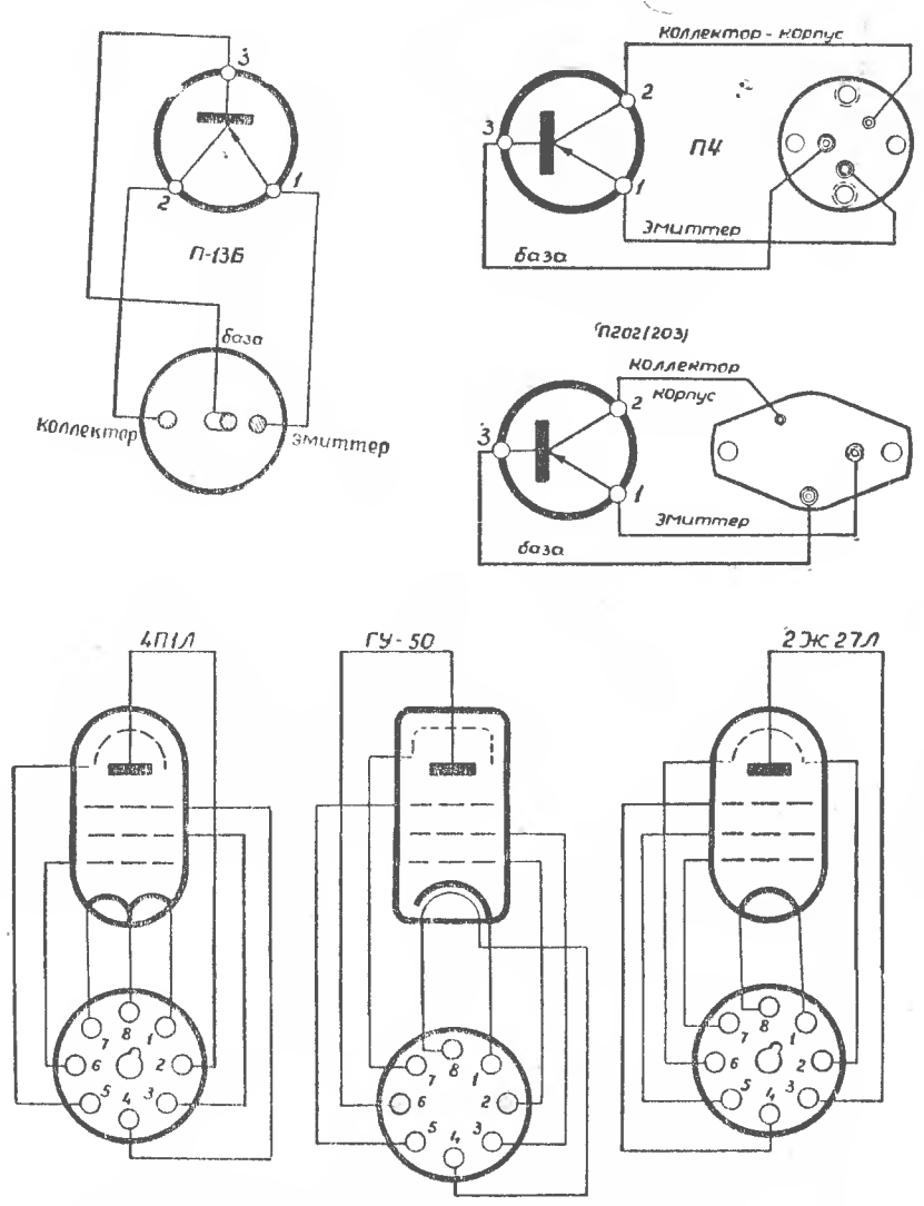
Цоколевка ламп и кристаллических триодов (вид снизу)
