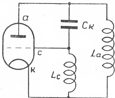
Упрощенная индуктивная трехчастотная схема плавного генератора без вспомогательных деталей.
