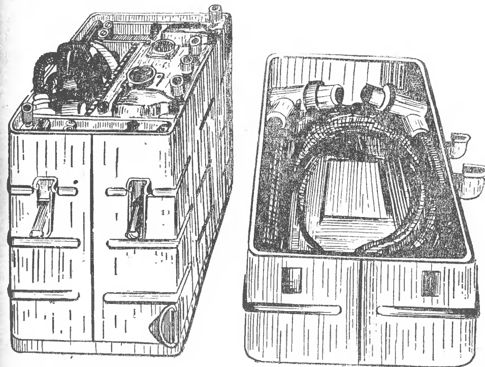
Рис. 17. Упаковка питания.
