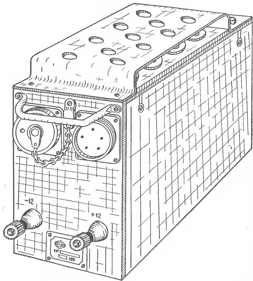
Рис. 18. Блок питания.
