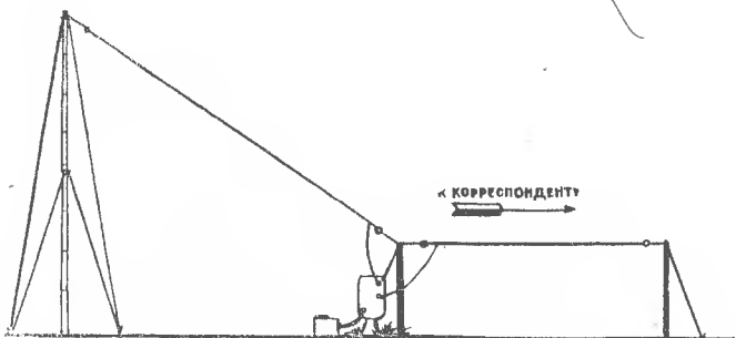
Установка антенны на специальной мачте.
