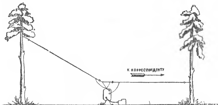
Установка антенны на естественных опорах.
