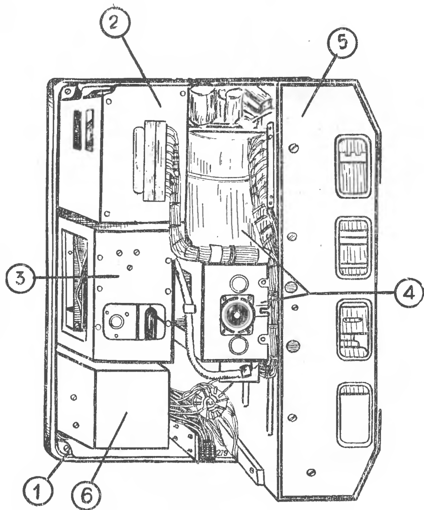
Рис. 16. Приемопередатчик (вид сзади).
