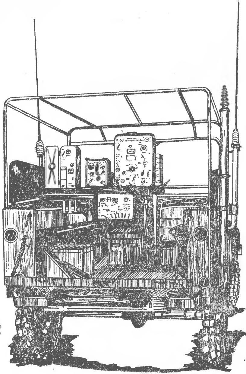
Рис. 20. Размещение радиостанции в автомобиле,
