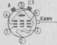
ПЕНТОД ГУ-81
