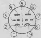
ДВОЙНОЙ ТРИОД 6X3II
