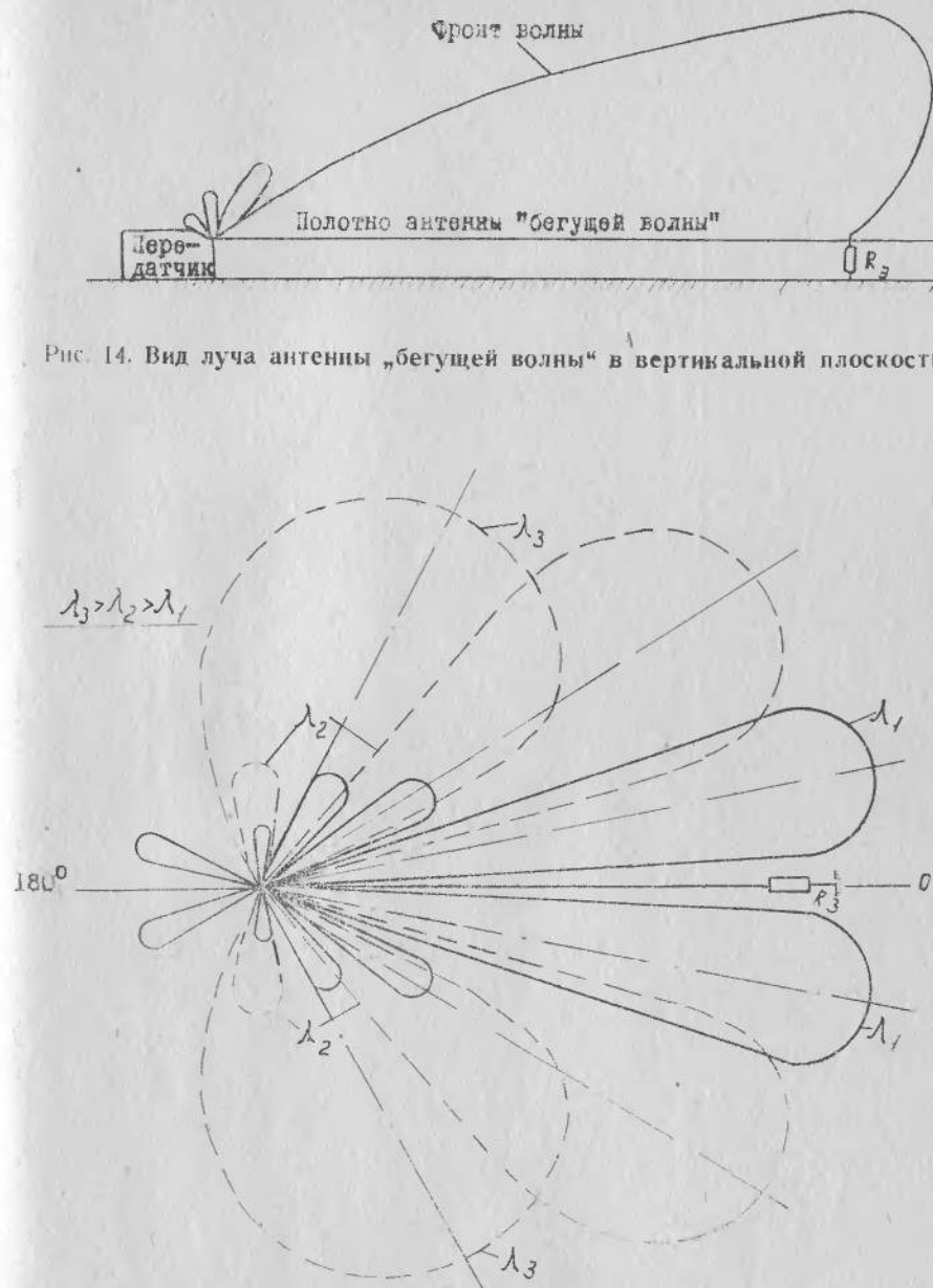
Рис. 15. Вид диаграммы направленности антенны "бегущей волны" в горизонтальной плоскости
