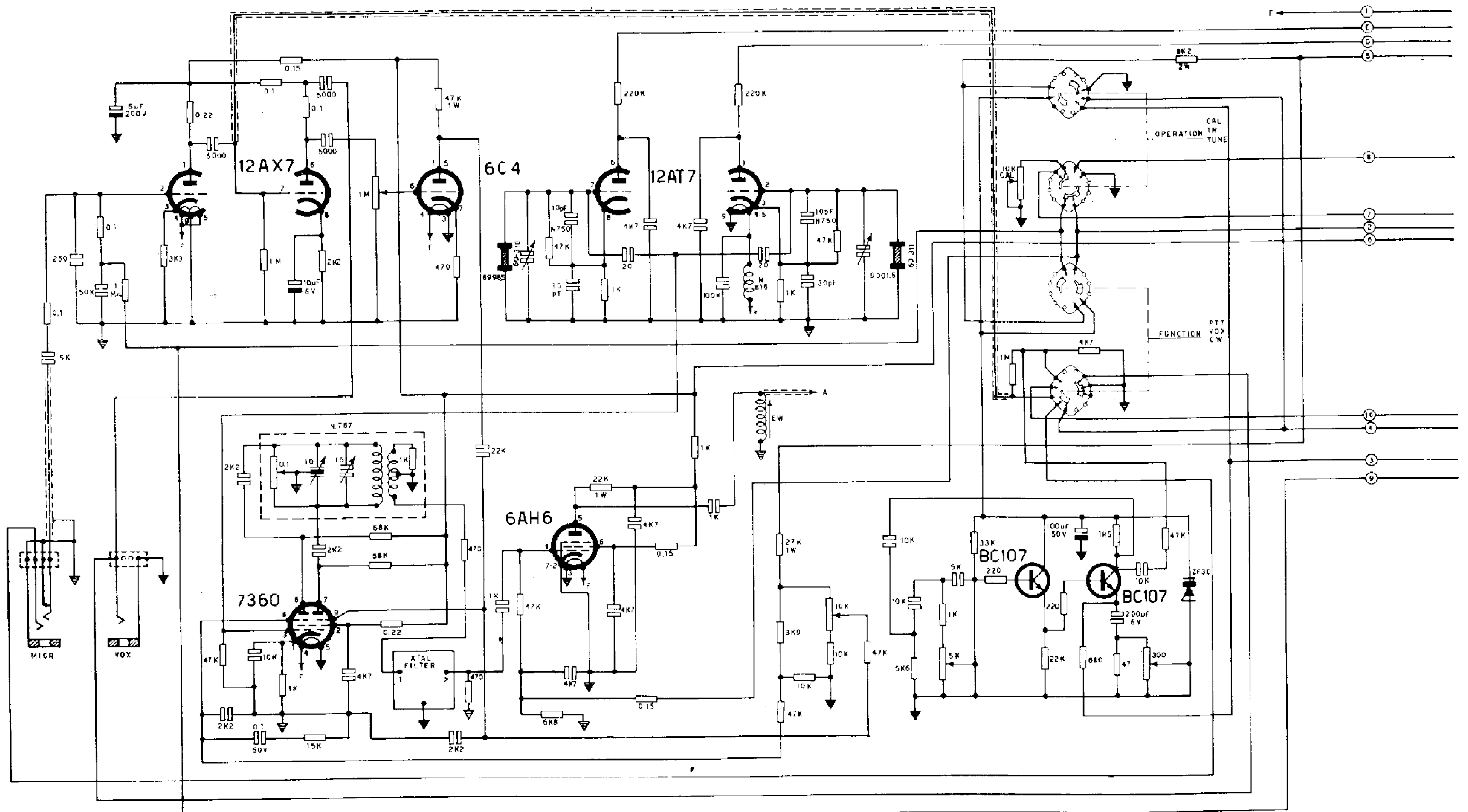
MODULATORE DEL TRASMETTITORE G 4/228 MK II
