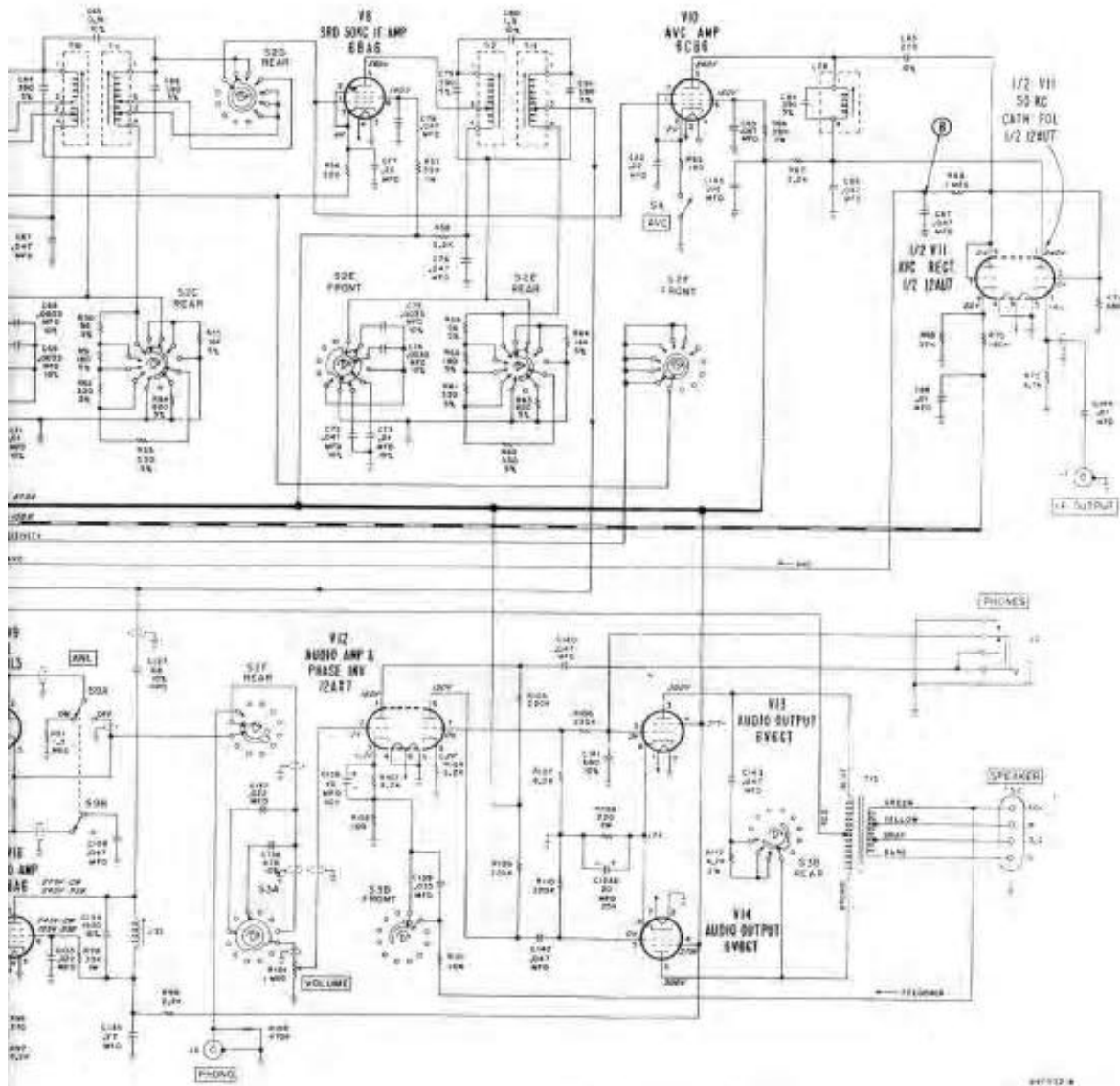
Fig. 20. Schematic Diagram
