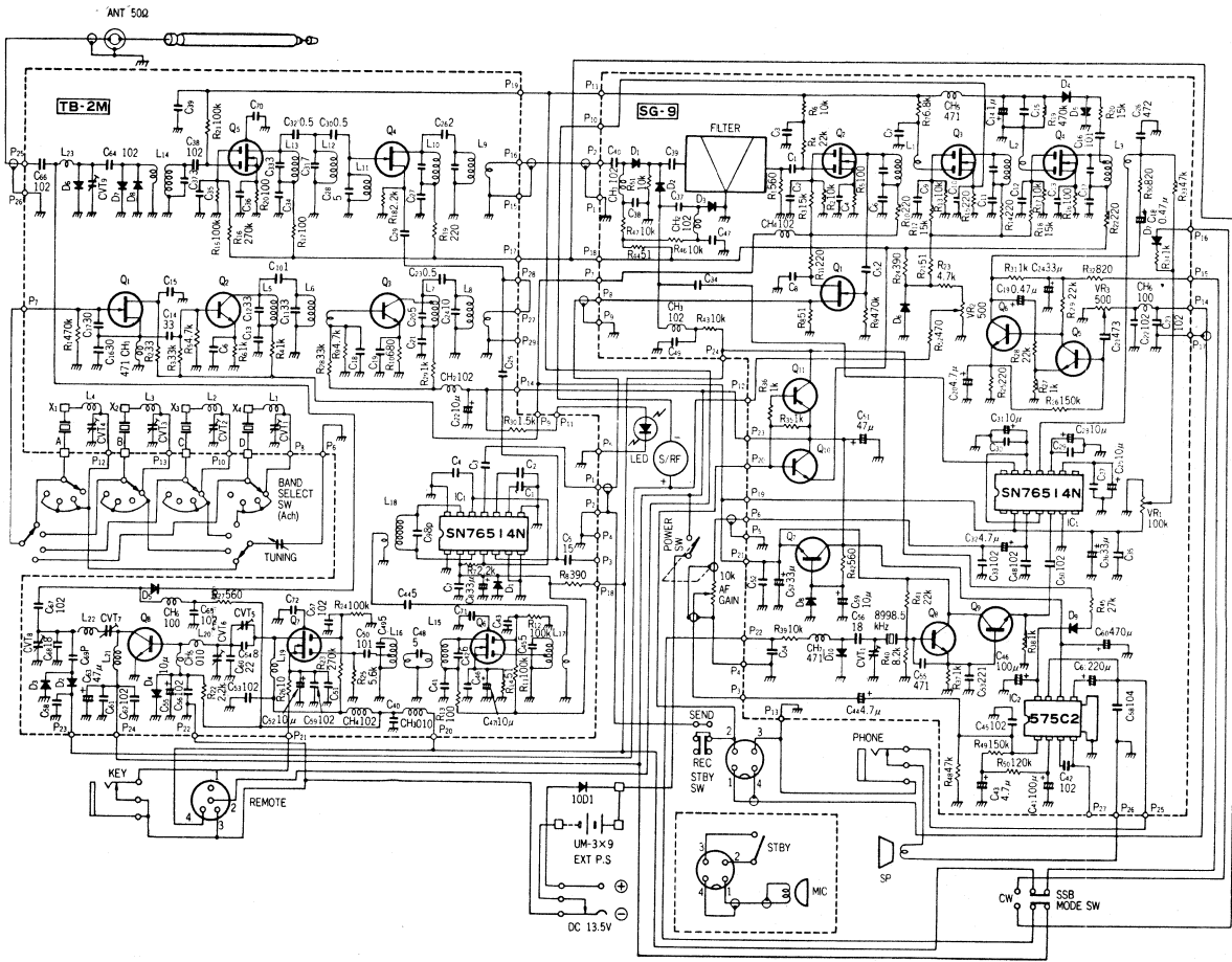
Gesamtschaltbild
