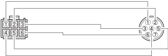
ピン挿入側より見た図
