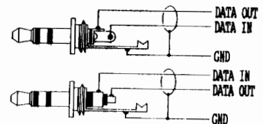
DATA IN/OUTプラグの接続
