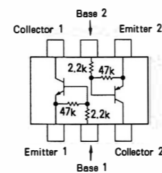
UMB10 (B10) (Q1006, 1010)
