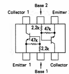
UMH10 (H10) (Q1011)
