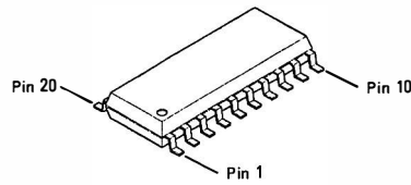
CM8880SIT-2 (Q101)
