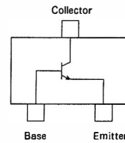
2SC2759 (U22) (Q305) 2SC3356 (R24) (Q301,303)
