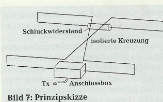
Bild 7: Prinzipskizze
