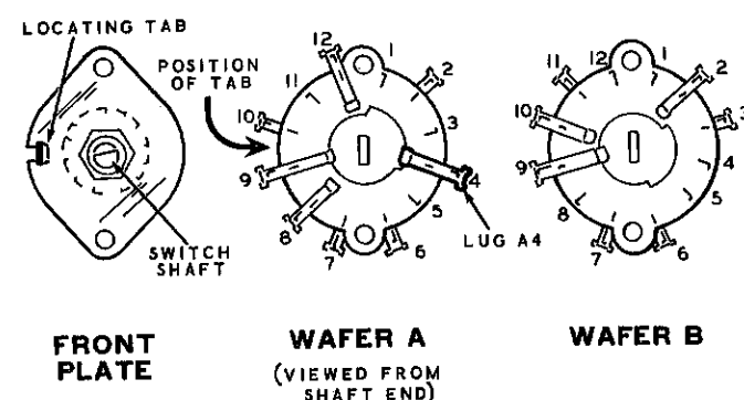
Detail 1A
