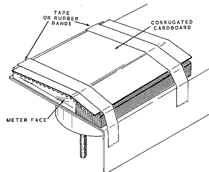
Detail 6F
