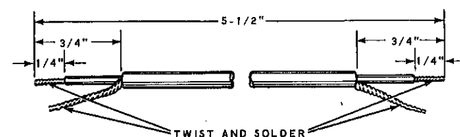
Detail 7E
