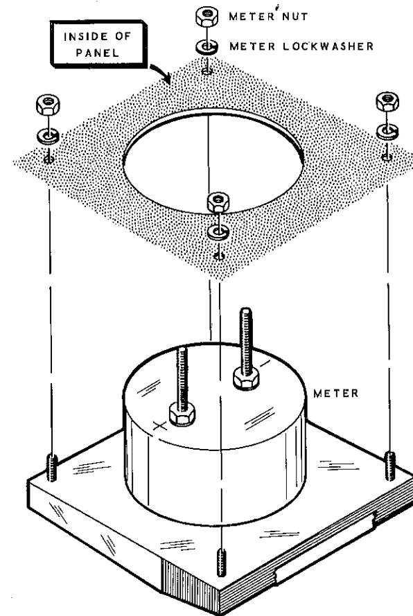
Detail 6E
