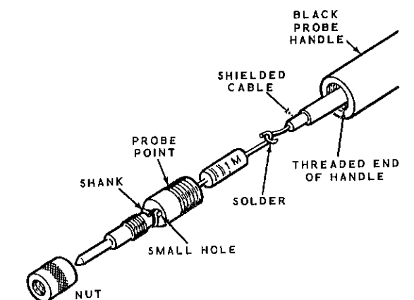
Detail 7D
