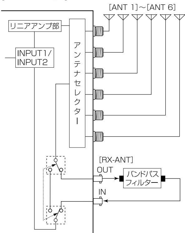
【RX-I/O回路概略図】
