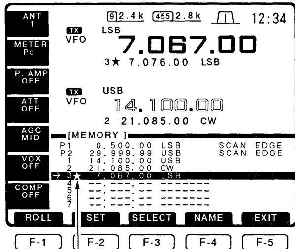
★マークが点灯し、セレクトチャンネルが指定される
