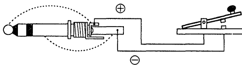
■電鍵・外部エレクトロニックキーヤーの接続
