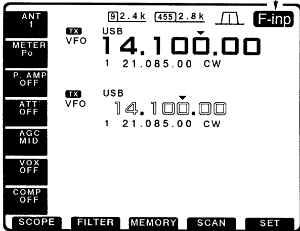
テンキー入力表示
