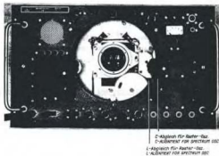
Bild 2 Einschub von vorn, Abdeckplatte und Skala abgenommen
