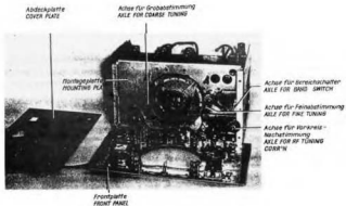
Bild 3 Einseh von vorn, Abdeckplatte und Frontplatte abgenommen
