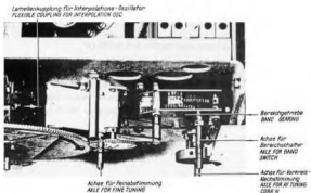
Bild 7 Bereichsgetriebe und Lamellenkupplung Fig. 7 BAND GEARING AND FLEXIBLE COUPLING
