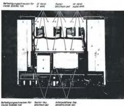
Bild 1 Einschub-Unterseite, Abdeckblech abgenommen
