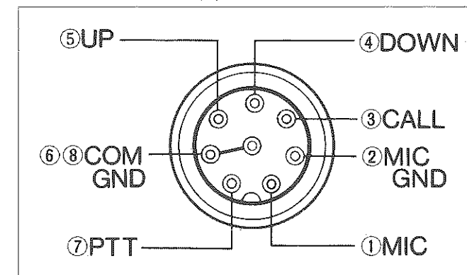
■マイクコネクター図
