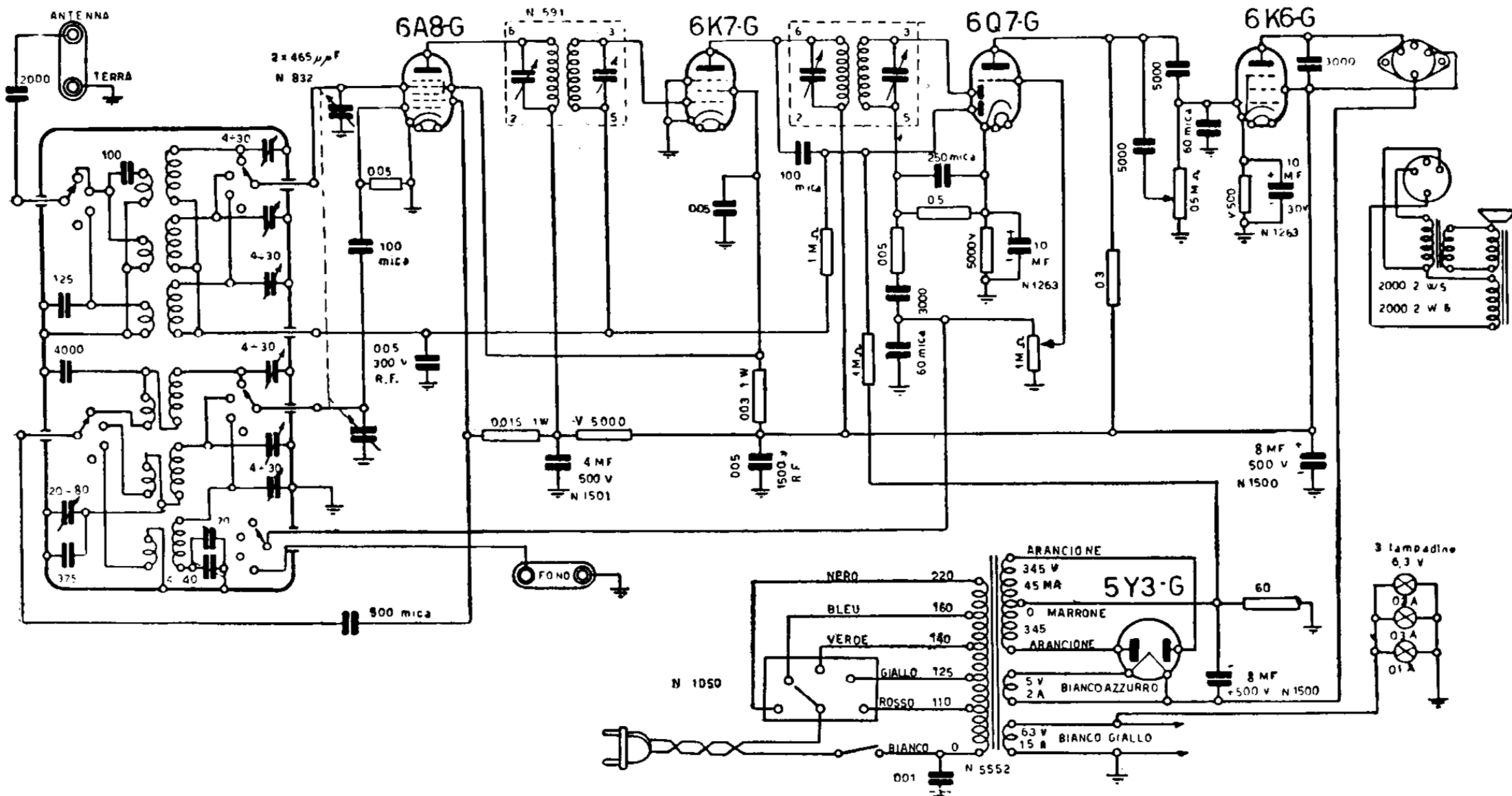
GELOSO. — Mod. G 50R. — Medie, corte e lunghe con AF 1911 A, e medie, corte e cortissime con 1912 A, scala 1776 Media frequenza: 467 kHz. — Produzione 1935-36.
